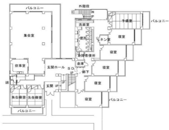
A棟1階
