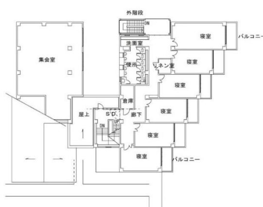
A棟2階
